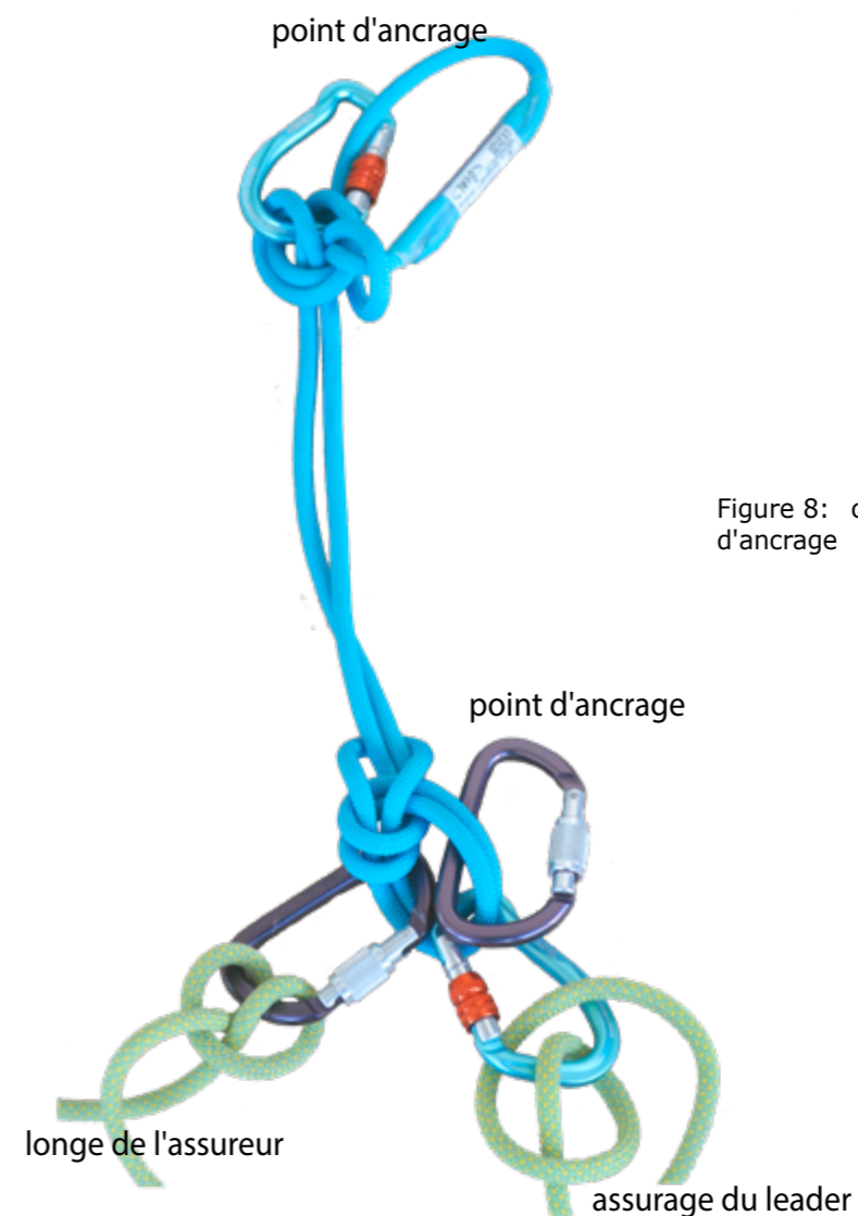
Figure 9: construction du relais avec deux points d'ancrage
